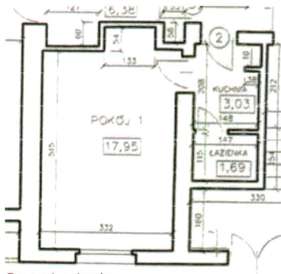
Rzut mieszkania
