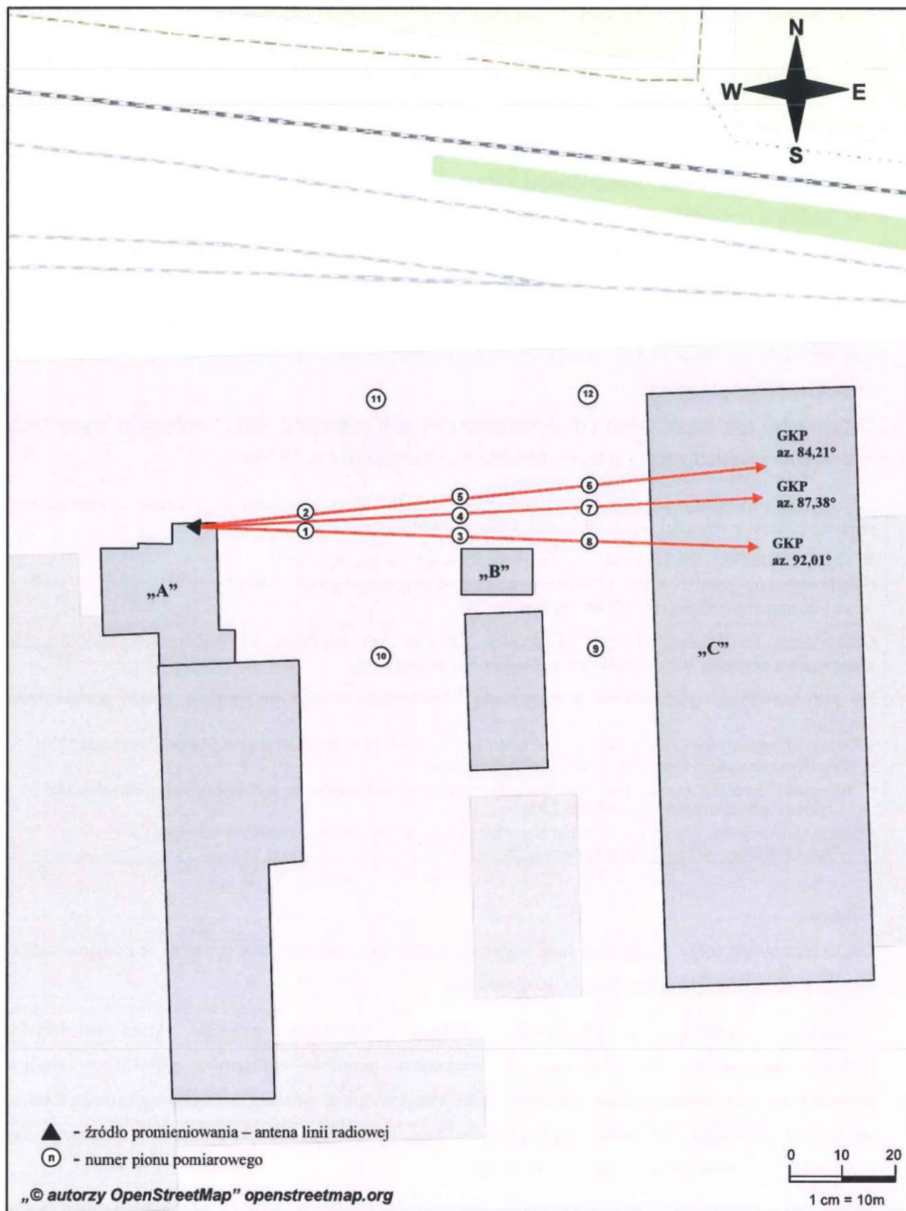
Rys. 1. Usytuowanie punktów i pionów pomiarowych w otoczeniu instalacji radiokomunikacyjnej Stacja Netia TYCYR009-TYCYM00008 Tychy, ul. Przemysłowa 55
