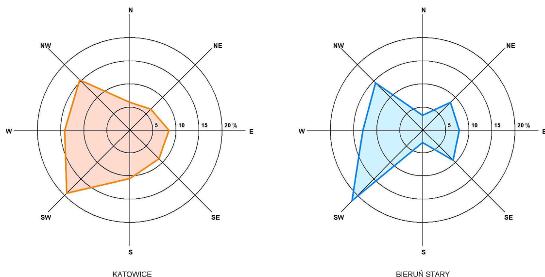
Rys. 1 Róże wiatrów dla stacji meteorologicznej Katowice – Muchowiec i posterunku meteorologicznego Bieruń Stary.
