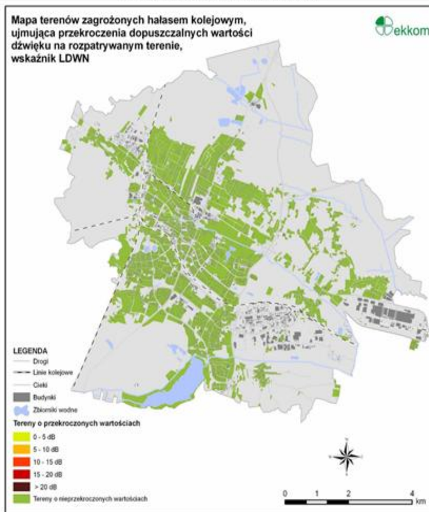
Rys. 4.5. Mapa terenów zagrożonych hałasem kolejowym na terenie Miasta Tychy - wskaźnik LDWN[38]
