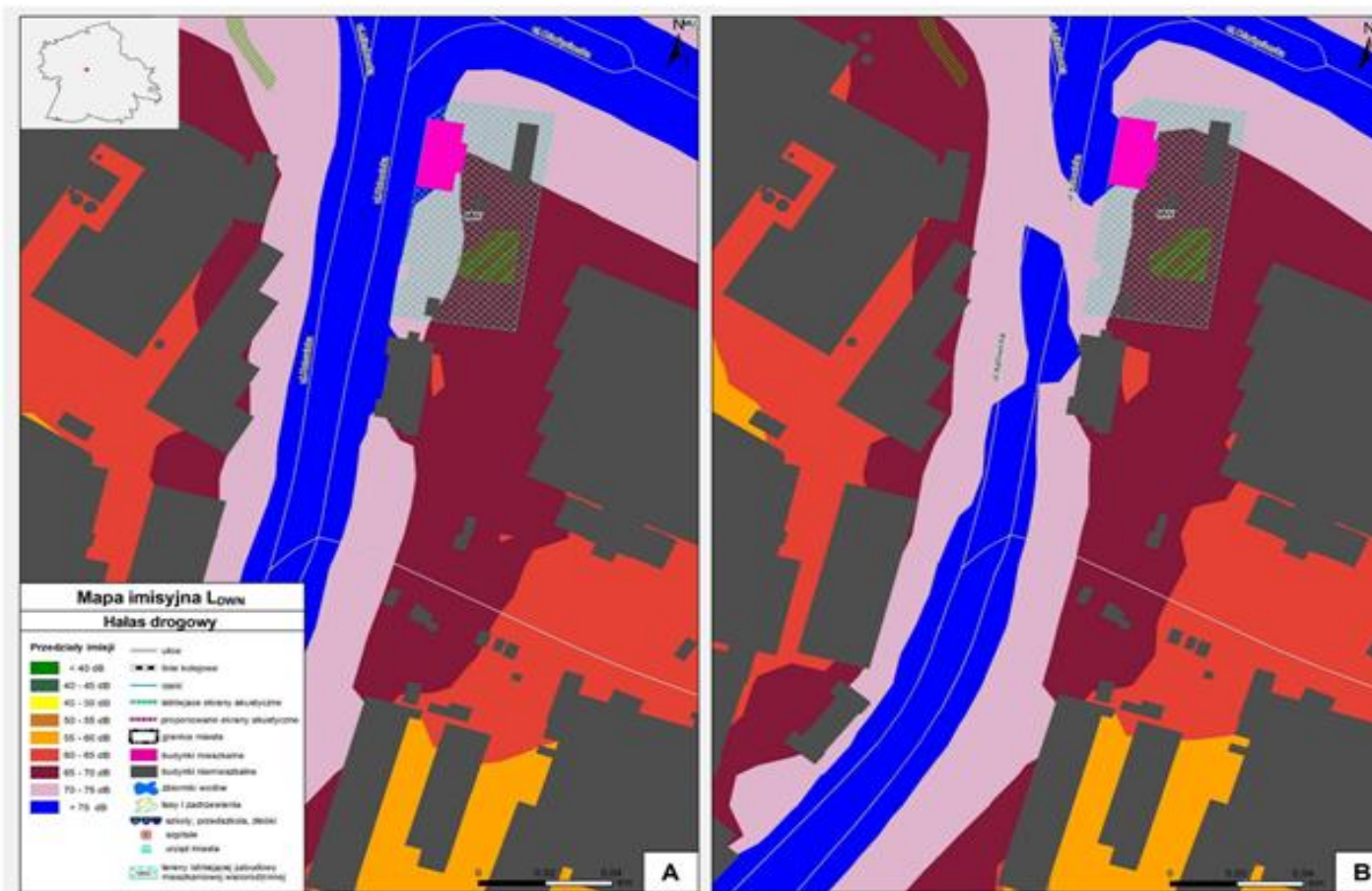
Rys. 2. Sytuacja przed (A) i po (B) zastosowaniu proponowanych działań ograniczających emisję hałasu do środowiska na ul. Katowickiej.
