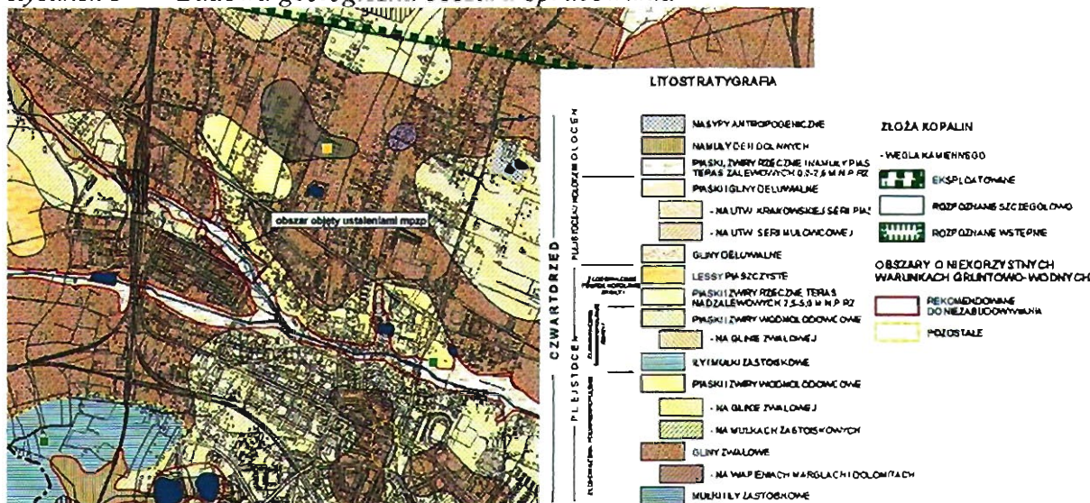
Rysunek 3 Budowa geologiczna obszaru opracowania
