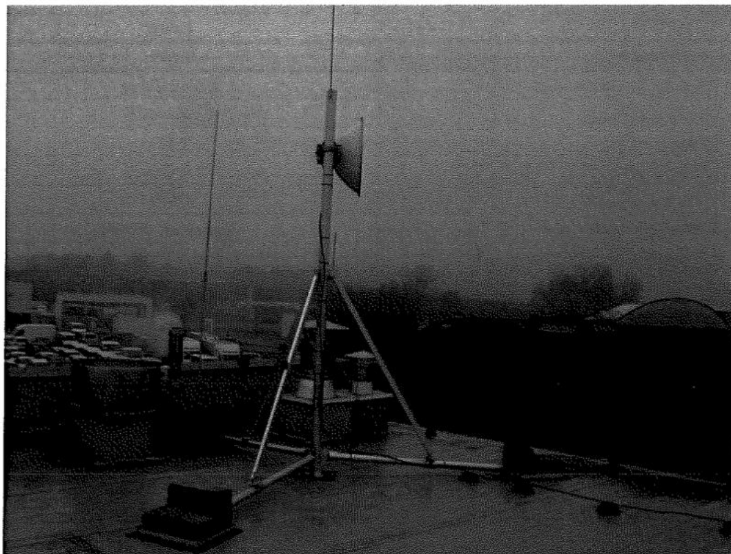
Fot. 1. OM Tychy / ul Strzelecka – widok anteny Emitel na dachu budynku
