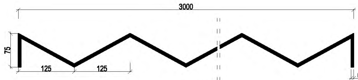
P-17 mini linia przystankowa
