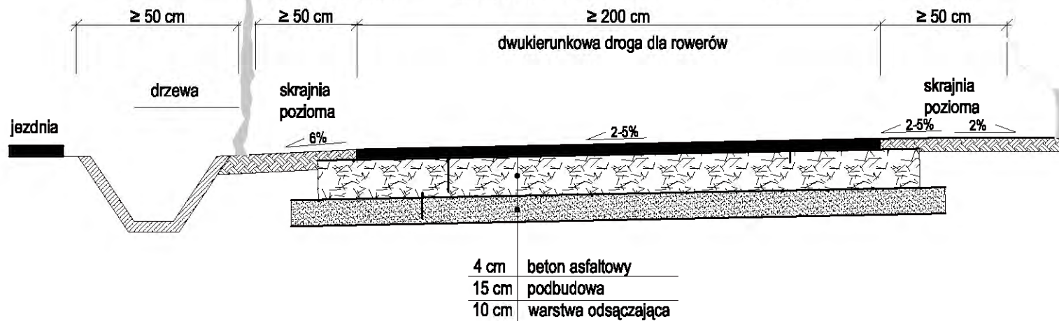
Dwukierunkowa droga dla rowerów na obszarze pozamiejskim bez obrzeży, ławy i oporu
