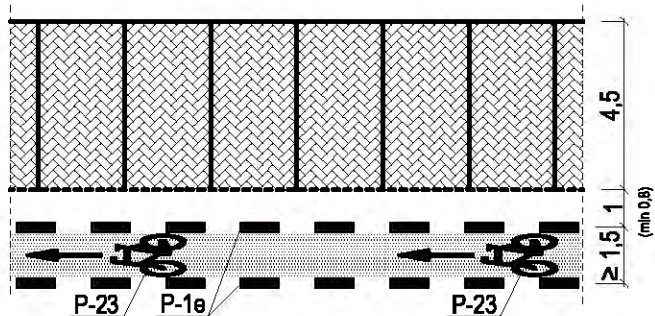
A - Parkowanie prostopadłe, zalecana opaska 1,0 m (min 0,8 m)
