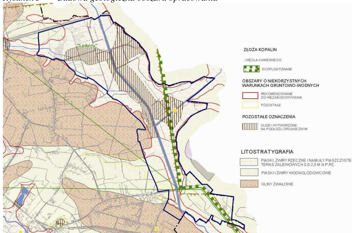
Rysunek 5 Budowa geologiczna obszaru opracowania
