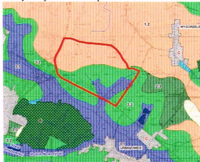
Rysunek 10 Topoklimaty w rejonie terenu opracowania
