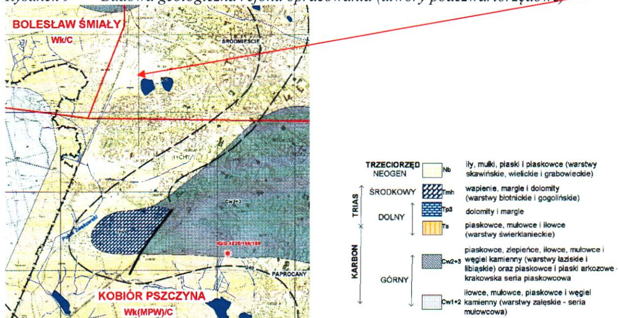
Rysunek 9 Budowa geologiczna rejonu opracowania (utwory podczwartorzędowe)
