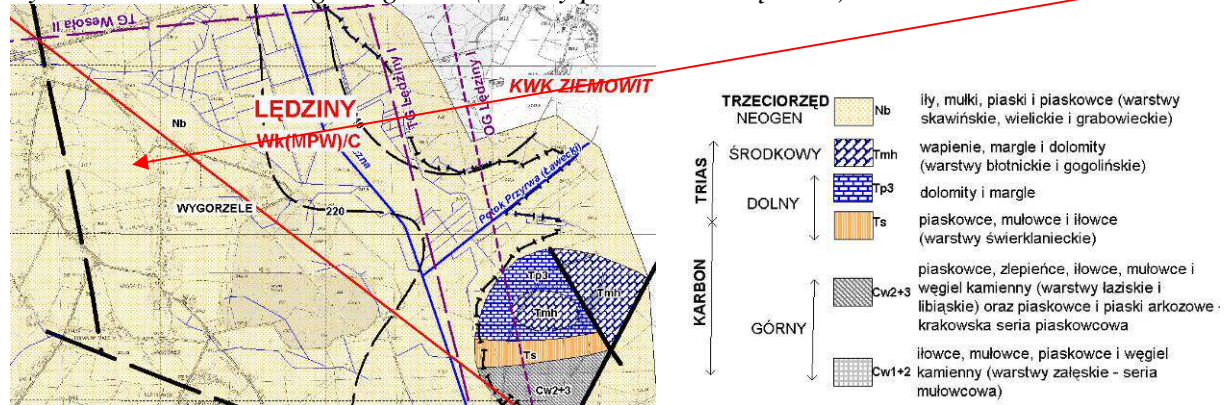
Rysunek 9 Budowa geologiczna (utwory podczwartorzędowe)
