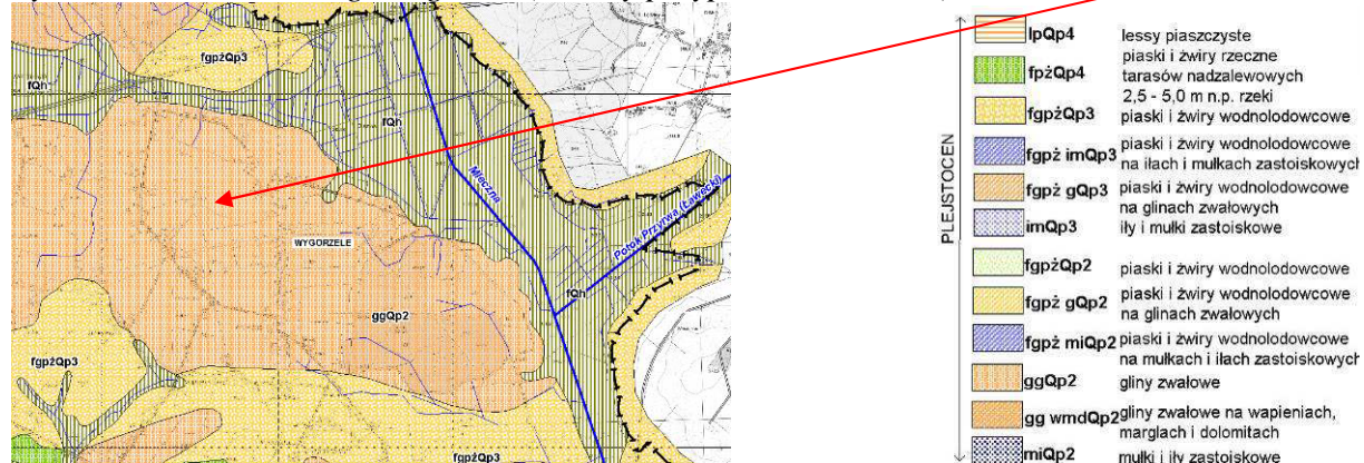
Rysunek 8 Budowa geologiczna (utwory przypowierzchniowe)
